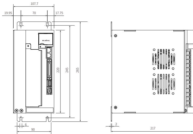
SE 4~5KW 驱动器安装尺寸图
