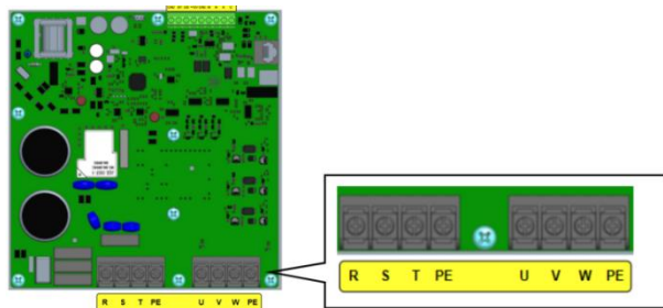
B2 机架主回路端子示意图 (4~5.5kW)
