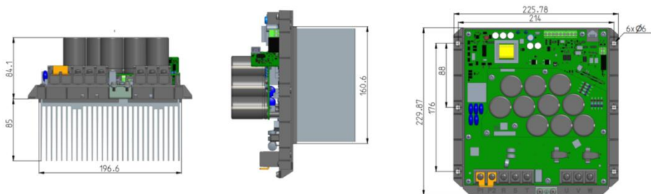
B4 机架安装尺寸示意图 (18.5~22kW)
