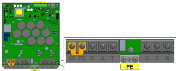
B4 机架主回路端子示意图（18.5~22kW）
