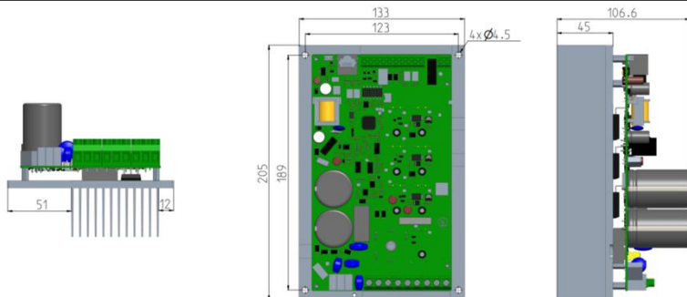
B1 机架安装尺寸示意图 (0.37~2.2kW)
