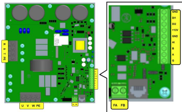
B3 机架控制回路端子示意图 (7.5~15kW)
