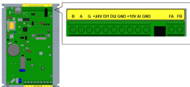
B1 机架控制回路端子示意图 (0.37~2.2kW)
