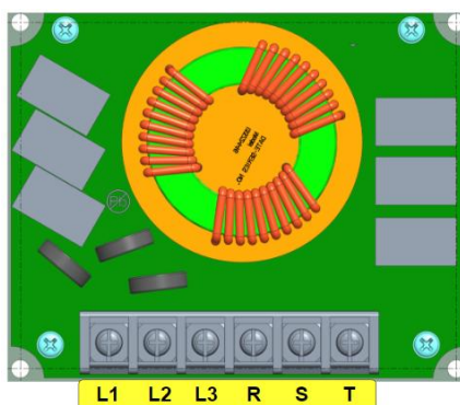
B4 机架选配 RFI 滤波板主回路端子示意图（18.5~22kW）
