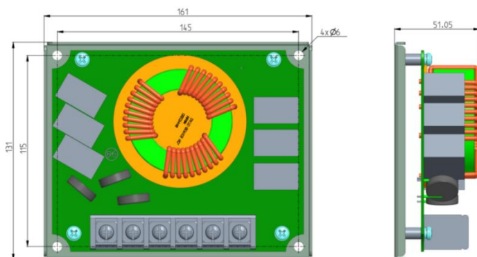
B4 机架外挂 RFI 滤波板安装尺寸示意图
