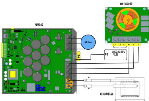
B4 机架选配外挂器件主回路连接示意图 (18.5~22kW)
