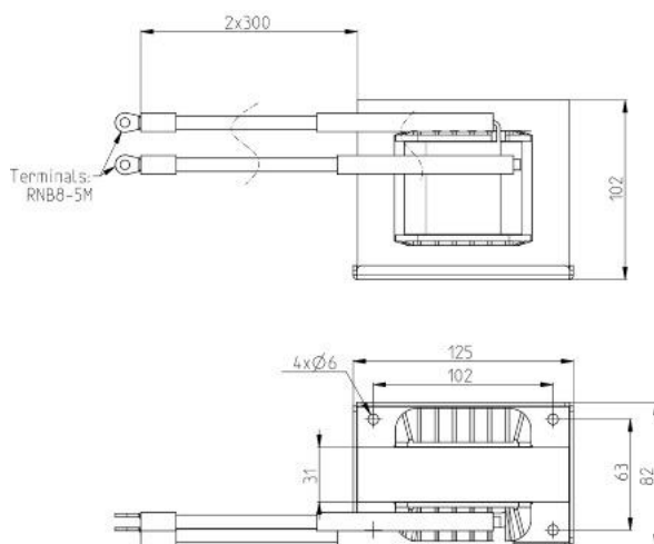
B4 机架外挂直流电抗器安装尺寸示意图
