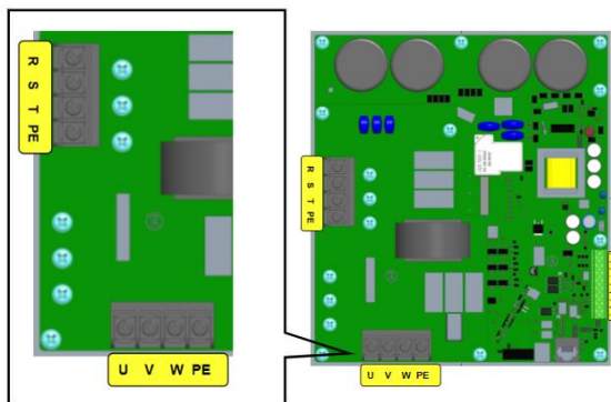
B3 机架主回路端子示意图 (7.5~15kW)
