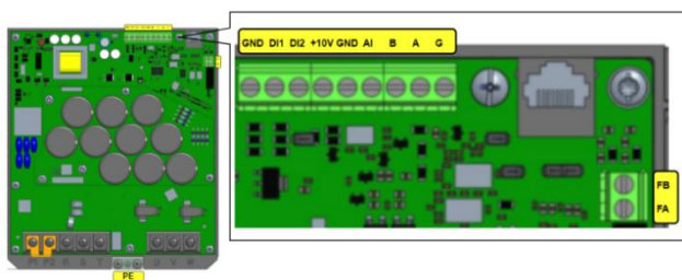
B4 机架控制回路端子示意图 (18.5~22kW)
