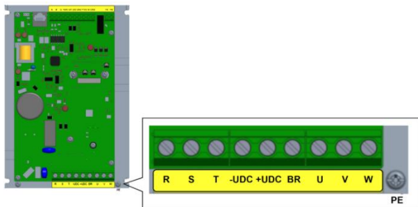
B1 机架主回路端子示意图 (0.37~2.2kW)
