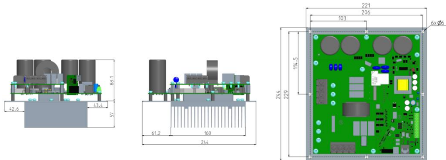
B3 机架安装尺寸示意图 (7.5~15kW)
