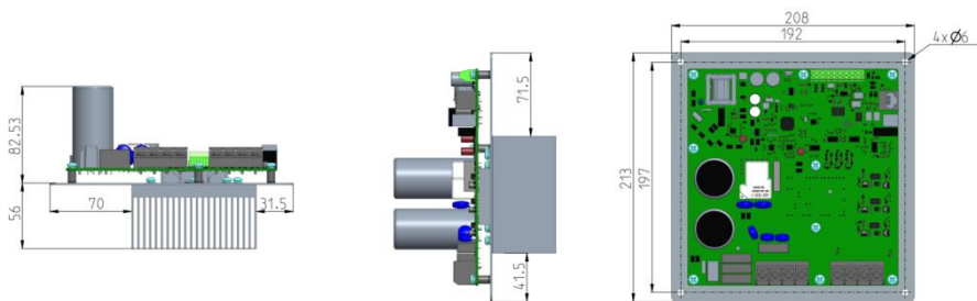
B2 机架安装尺寸示意图 (4~5.5kW)
