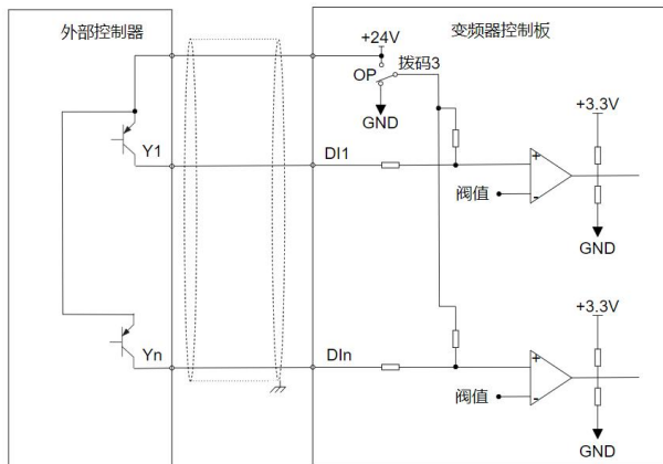
开路集电极 PNP 接线方式
