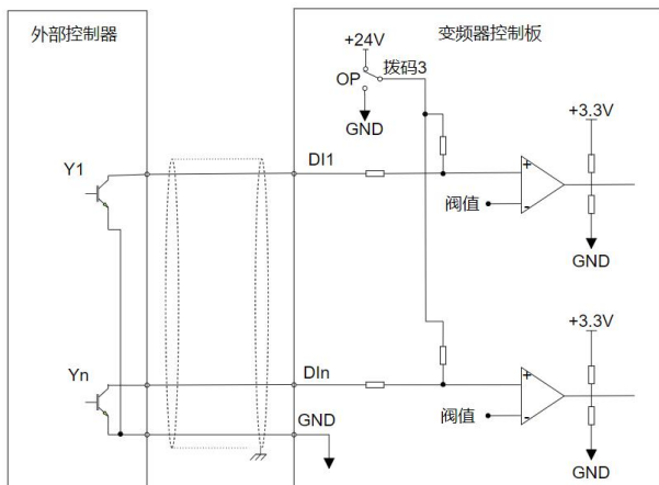
开路集电极 NPN 接线方式
