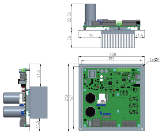
B2机架安装尺寸示意图 (4-5.5kW)
