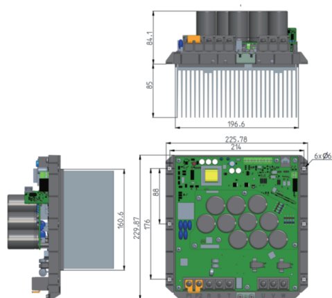
B4机架安装尺寸示意图 (18.5-22kW)
