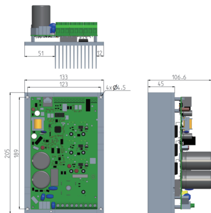
B1机架安装尺寸示意图 (0.37-2.2kW)
