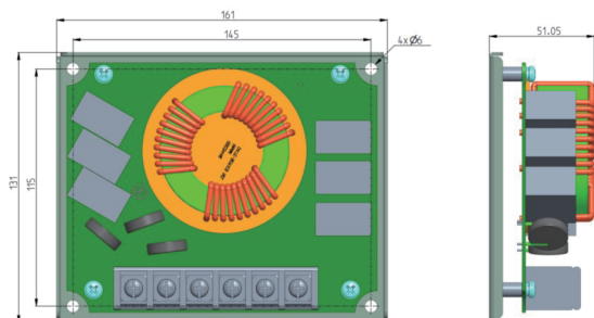
B4机架外挂RFI滤波板安装尺寸示意图
