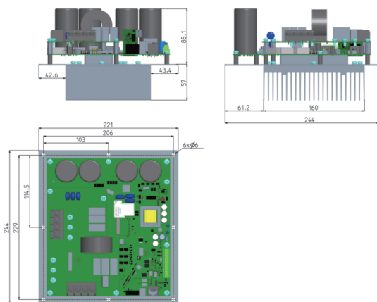
B3机架安装尺寸示意图 (7.5-15kW)
