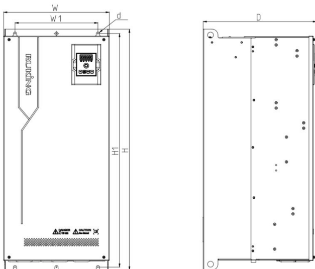
A5~A8 机架安装尺寸图
