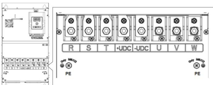
A5~10 机架主回路示意图 (30~560kW)
