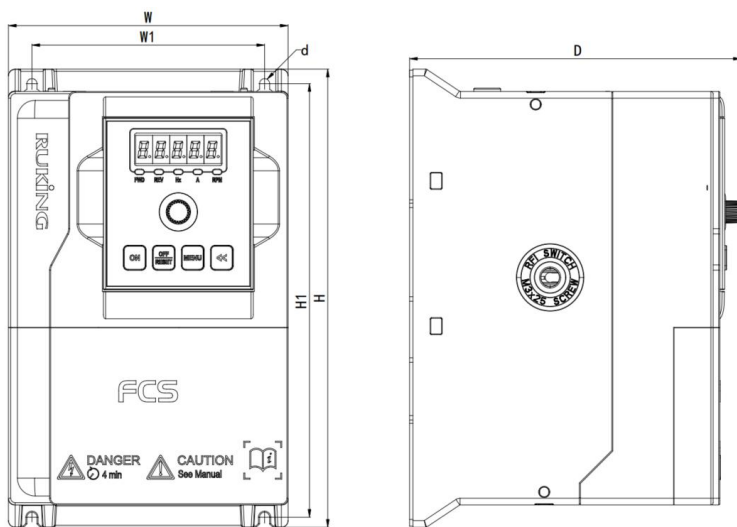
A0~A4 机架安装尺寸图
